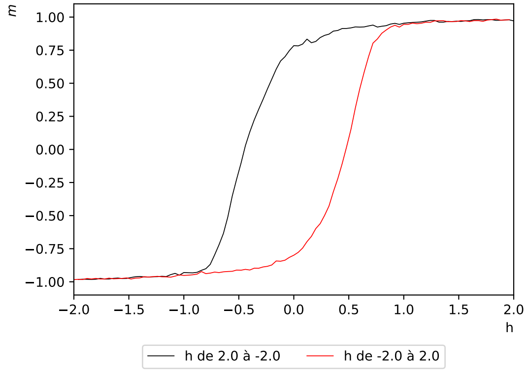
Hystérésis de l'aimantation - réseau de taille L=64 - champ magnétique d'amplitude h=2 à T=2.5
